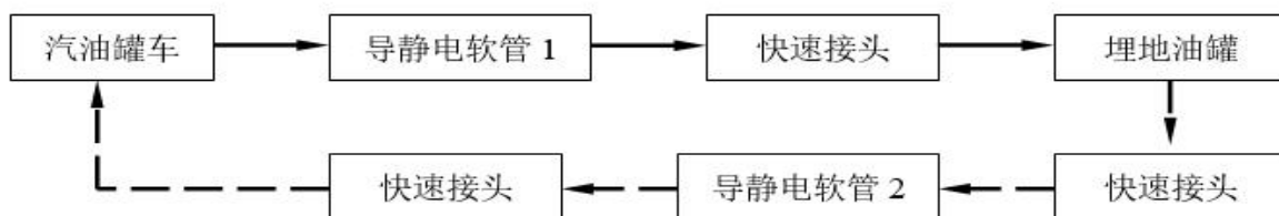
图 2.5-1 汽油卸油工艺流程示意简图
