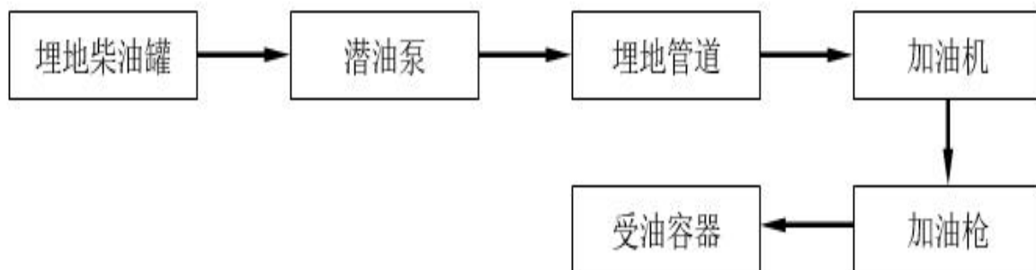
图 2.5-4 柴油加油工艺流程图示意简图
