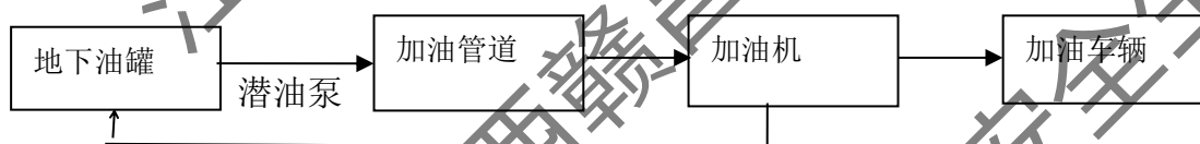
柴油加油工艺流程图
